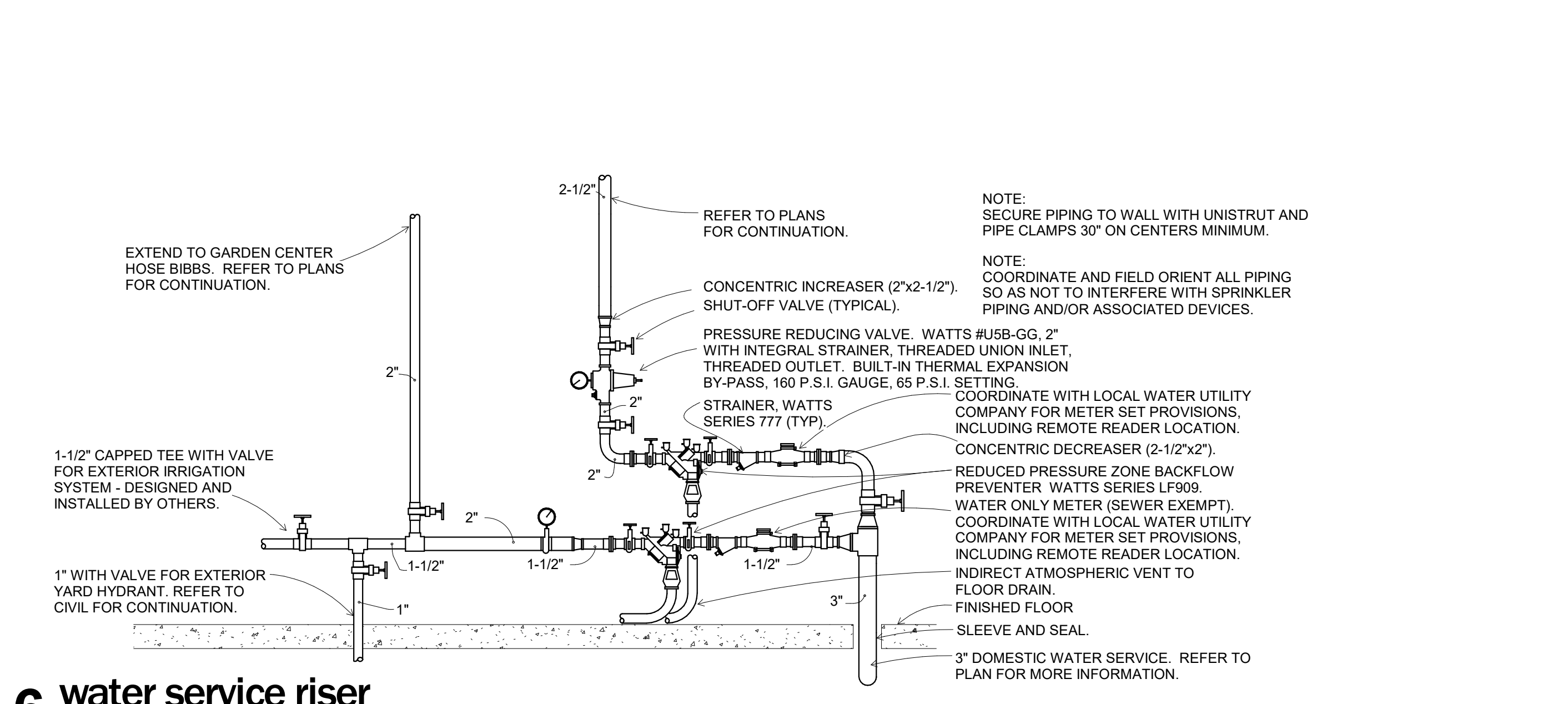
6 water service riser SCALE | N.T.S.
