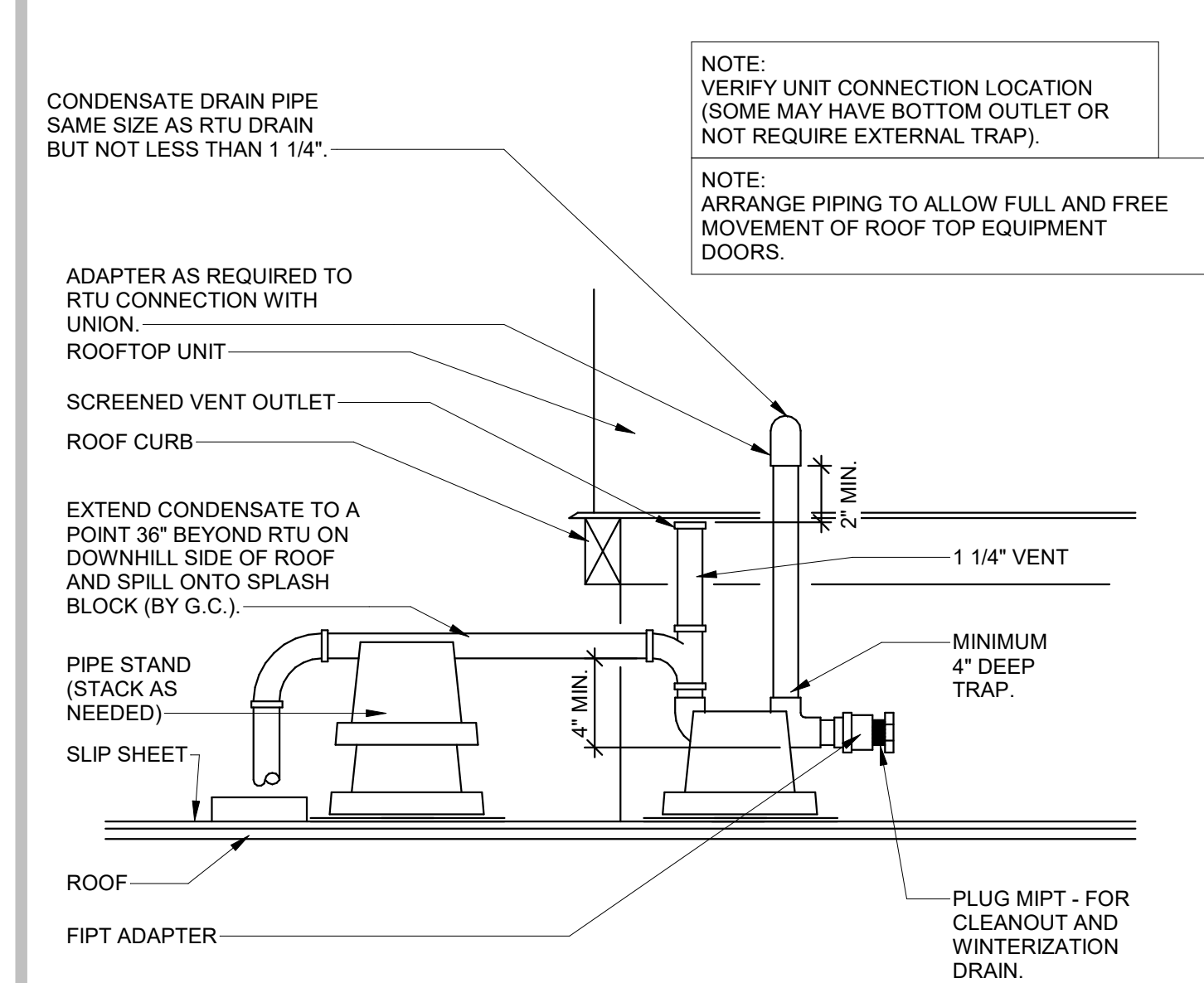
5 RTU condensate drain SCALE | N.T.S.
