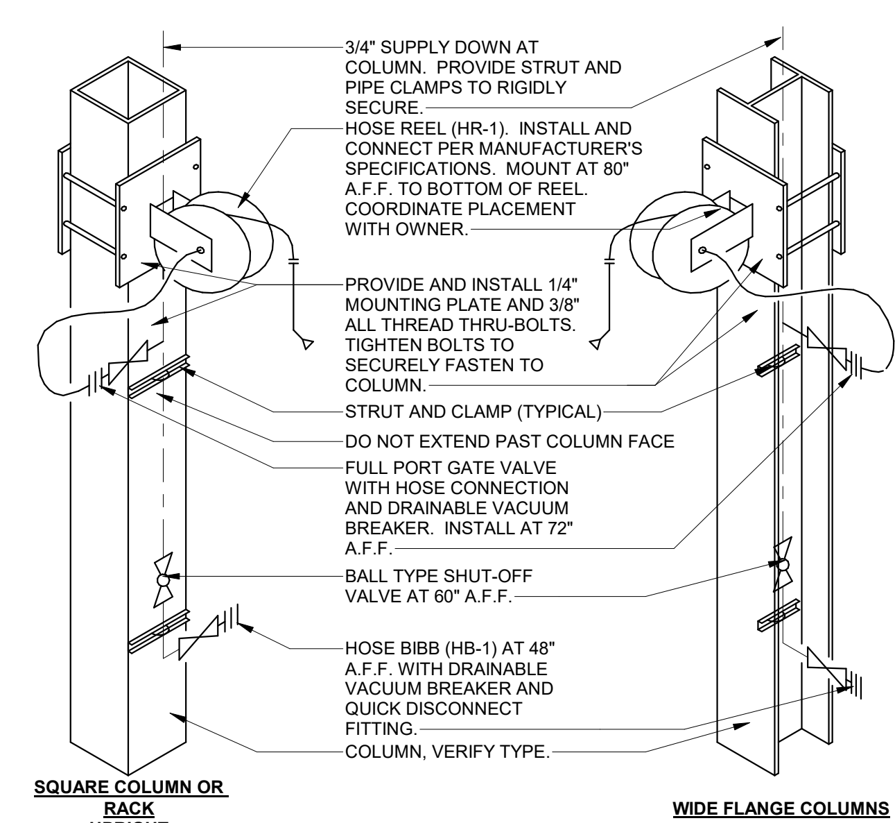
3 garden area hose reel SCALE | N.T.S.
