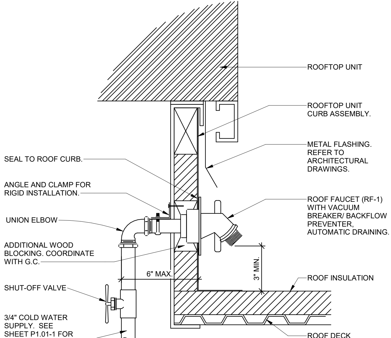
2 roof faucet (RF-1) SCALE | N.T.S.
