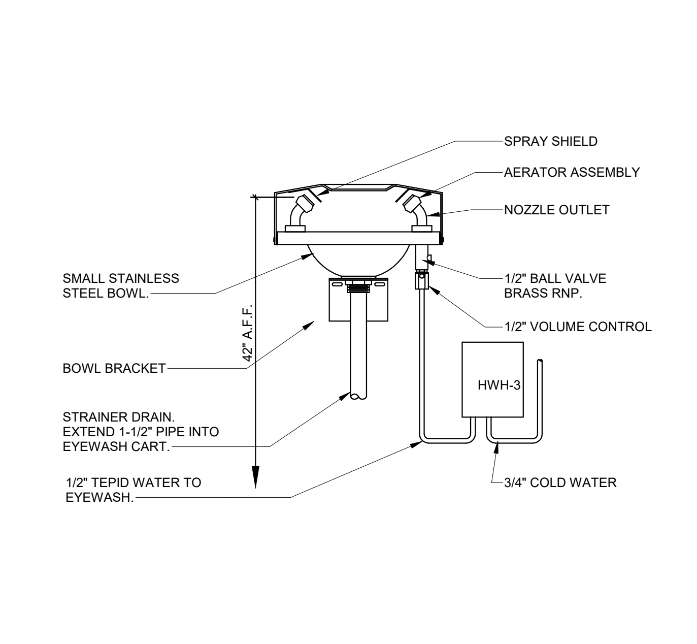
8 emergency eyewash SCALE | N.T.S.
